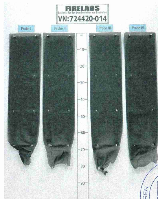
Bild 28 Aussehen des Probekörpers nach dem Brandversuch
