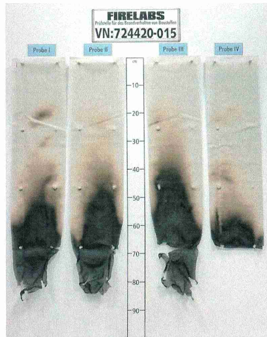
Bild 30 Aussehen des Probekörpers nach dem Brandversuch
