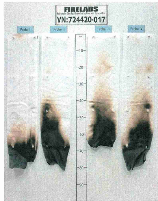
Bild 34 Aussehen des Probekörpers nach dem Brandversuch
