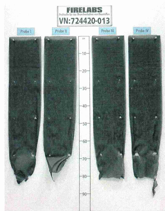
Bild 26 Aussehen des Probekörpers nach dem Brandversuch
