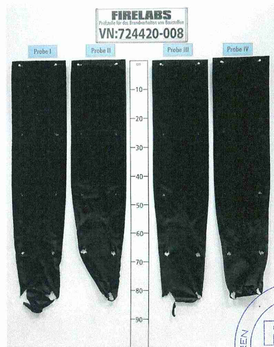
Bild 16 Aussehen des Probekörpers nach dem Brandversuch
