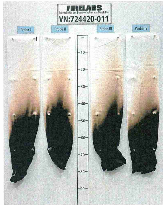
Bild 22 Aussehen des Probekörpers nach dem Brandversuch
