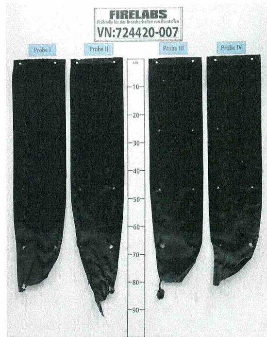
Bild 14 Aussehen des Probekörpers nach dem Brandversuch
