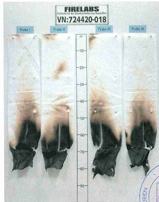
Bild 36 Aussehen des Probekörpers nach dem Brandversuch
