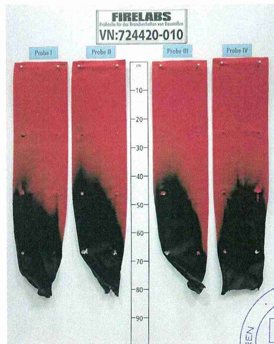
Bild 20 Aussehen des Probekörpers nach dem Brandversuch
