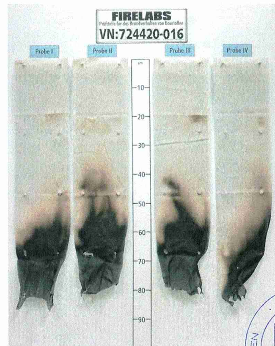
Bild 32 Aussehen des Probekörpers nach dem Brandversuch
