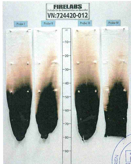
Bild 24 Aussehen des Probekörpers nach dem Brandversuch
